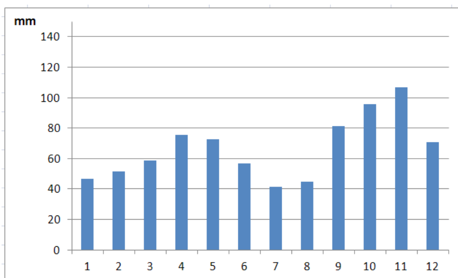
Figura 24. Diagramma delle precipitazioni medie mensili relativo alla stazione meteorologica di Arezzo-Molin Bianco nel periodo 1961-2010
