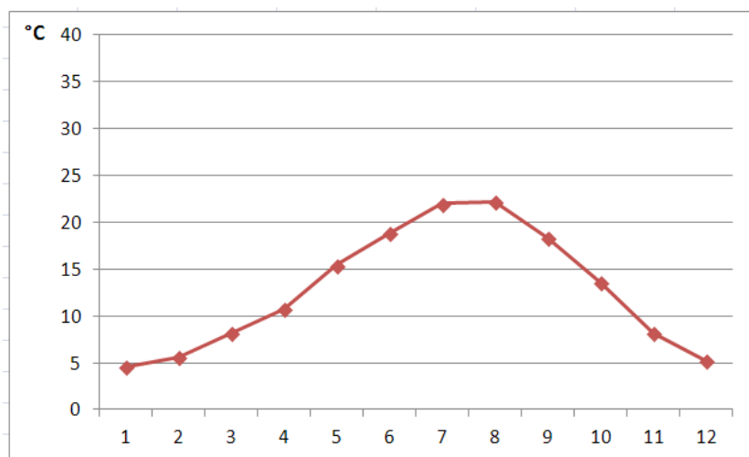
Figura 23. Diagramma delle temperature medie mensili relativo alla stazione meteorologica di Arezzo-Molin Bianco nel periodo 1961-2010
